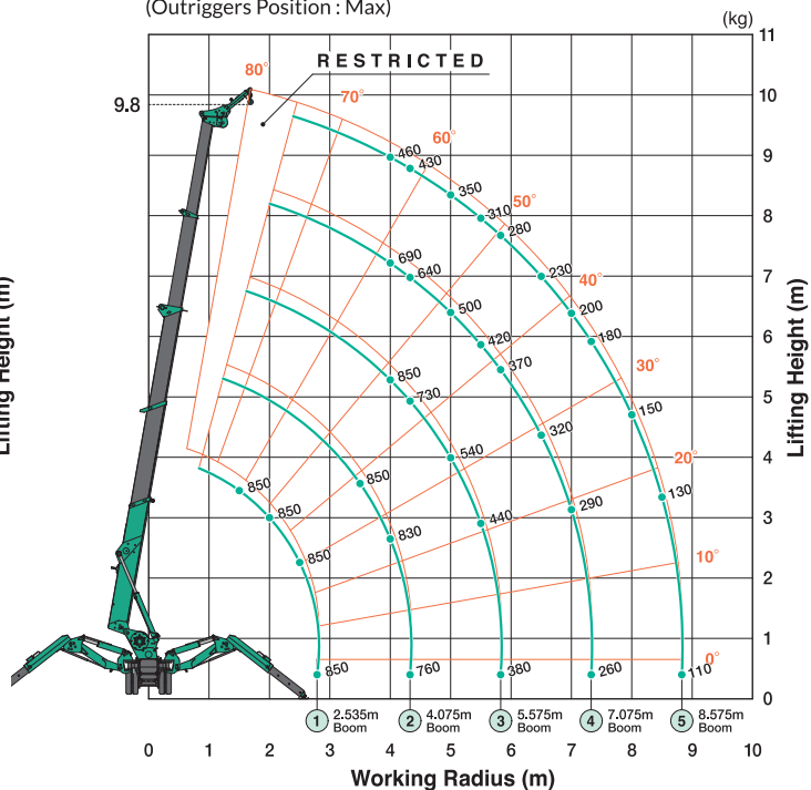
850kg Searcher Hook Offset Position : SH2 (Outriggers Position : Max)
